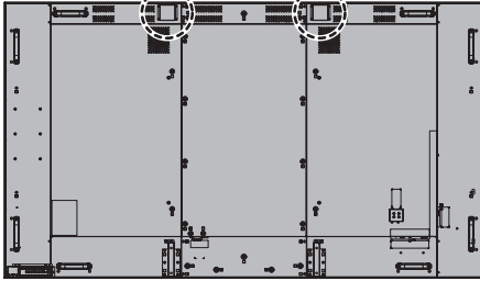
Ringschrauben (handelsüblich)- Befestigungspositionen
