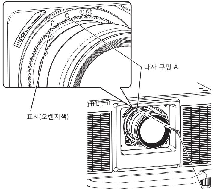
렌즈 고정 나사
