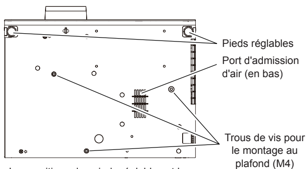
Les positions des pieds réglables et les trous de vis pour le montage au plafond
