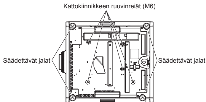
Kattokiinnikkeen ja säädettävien jalkojen ruuvireiän sijainnit
