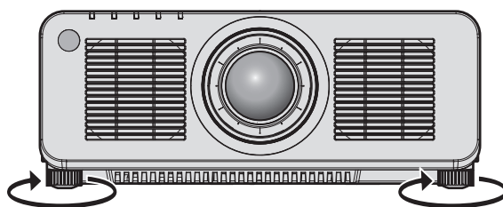
Rango ajustable máximo Pie ajustable: 30 mm (1-3/16") cada uno
