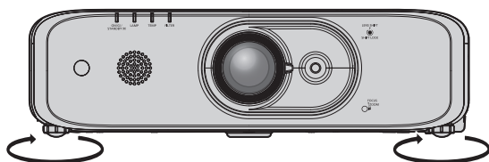
Rango ajustable máximo Pies ajustables: 23 mm (29/32") cada uno
