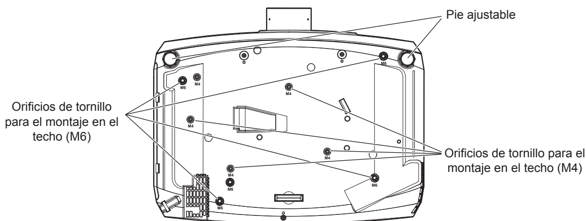
Posiciones de los orificios de tornillo para el montaje en el techo y uso de pie ajustable
