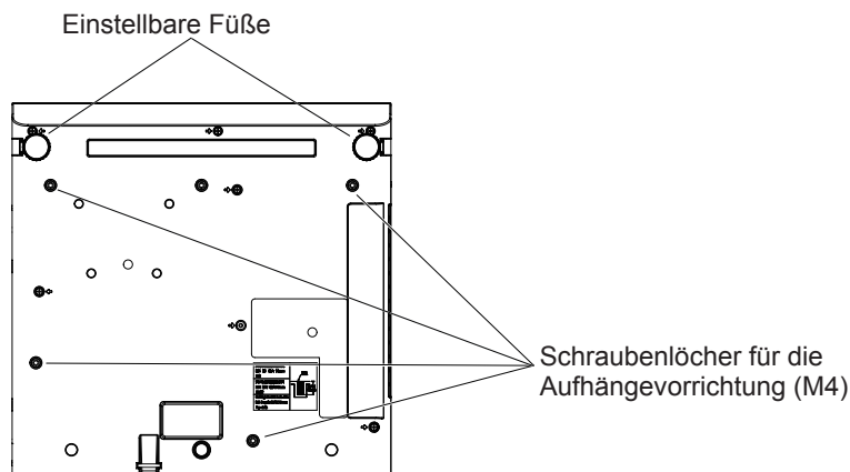
Positionen der Schraubenlöcher für die Aufhängevorrichtung und der einstellbaren Füße
