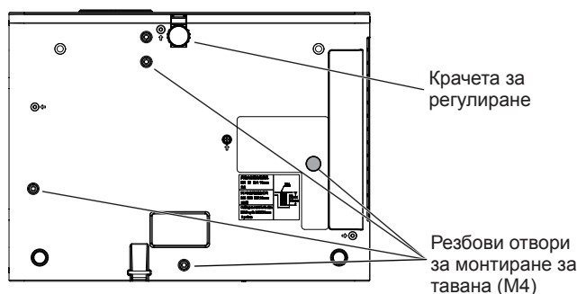
Позиции на отворите за винтове за таванен монтаж и крачета за регулиране
