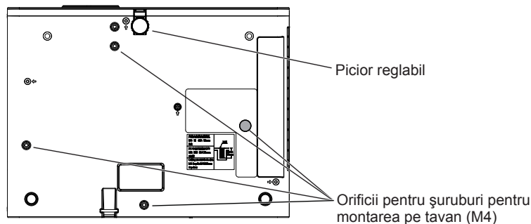
Pozițiile găurilor filetate pentru instalarea pe tavan și a piciorului reglabil
