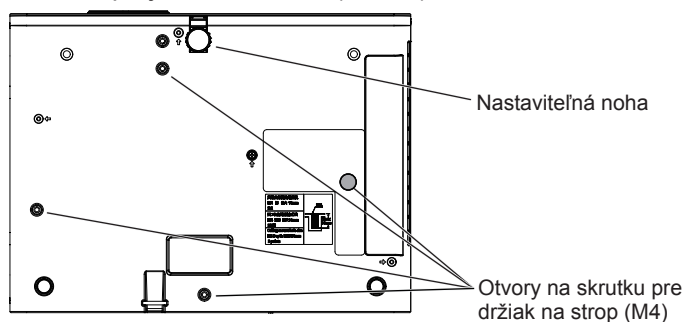
Polohy otvorov pre skrutky pre stropné držiaky a nastaviteľnú nohu
