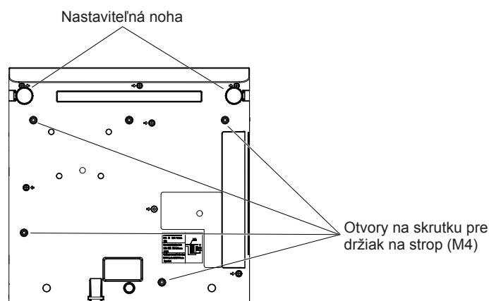
Umiestnenie otvorov na skrutku pre držiak na strop a nastaviteľnú nohu
