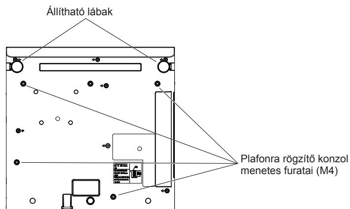
A plafonra rögzítő konzol menetes furatainak és az állítható lábak elhelyezkedése
