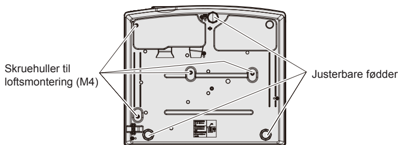
Skruenhullernes positioner til loftsmontering og justerbare fødder
