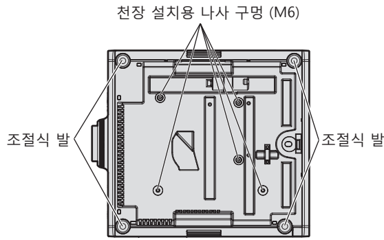
천장 설치용 나사 구멍과 조절식 발의 위치
