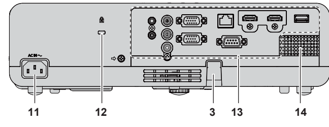
■ Вид сзади
