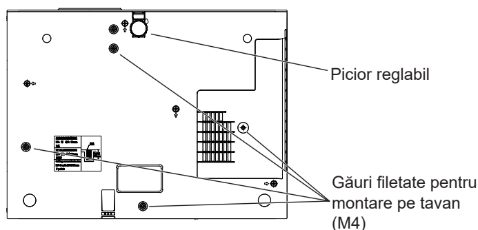
Pozițiile găurilor filetate pentru instalarea pe tavan și a picior reglabil
