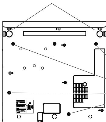
Polohy otvory šroubů pro stropní držák a nastavitelné patky
