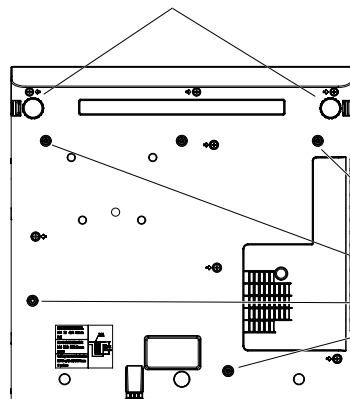
Placering af skruehullerne til loftsbeslaget samt justerbare fodder
