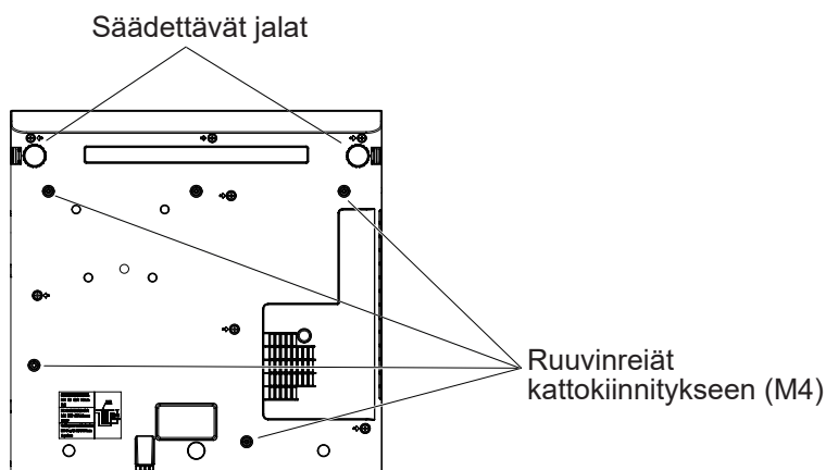
Ruuvinreikien sijainnit kattokiinnitykseen ja säädettävät jalat
