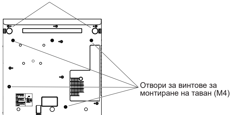
Позиции на отворите за винтове за монтиране на тавана и крачета за регулиране
