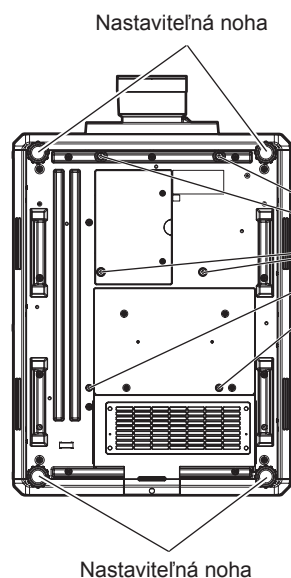
Umiestnenie otvorov na skrutku na upevnenie projektora a nastaviteľnú nohu
