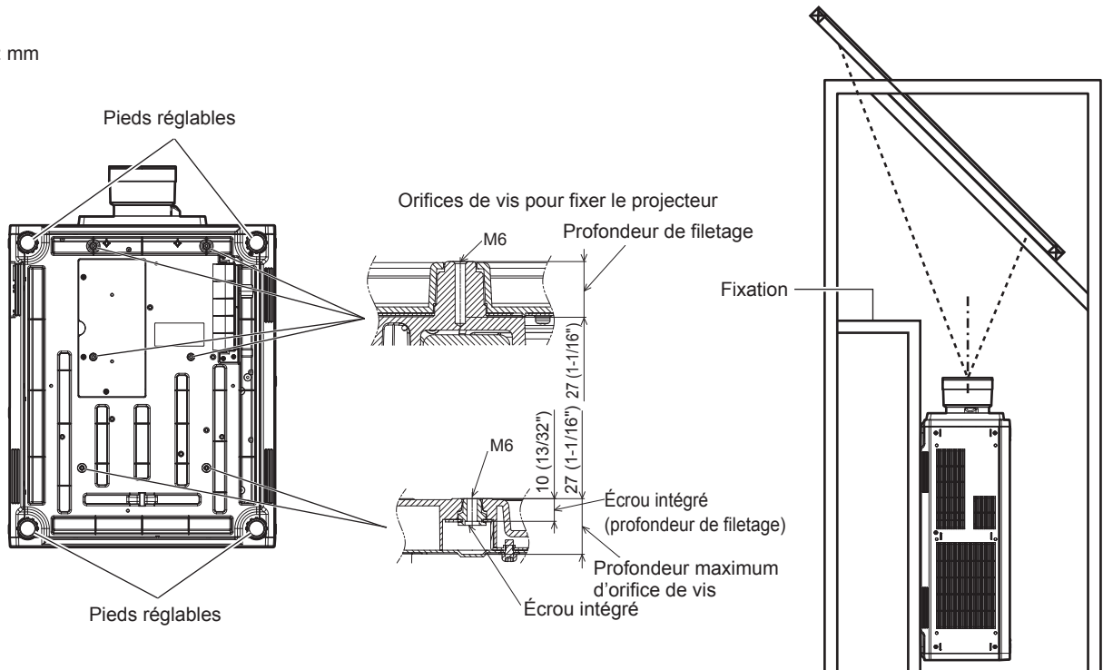
Positions des orifices de vis pour fixer le projecteur et les pieds réglables
