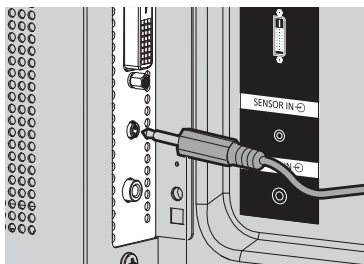
4-πολικό μικροσκοπικό καλώδιο φως
