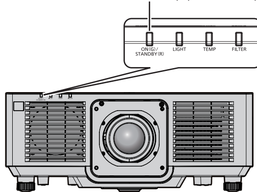
Indicatore di alimentazione <ON (G)/STANDBY (R)>
