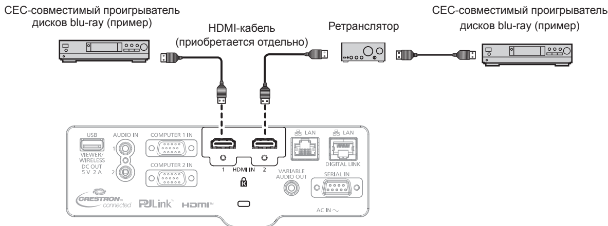
Пример подключения с CEC-совместимым устройством
