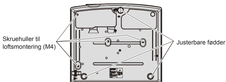
Skruehullernes positioner til loftsmontering og justerbare fødder
