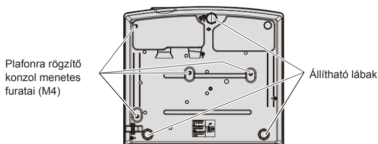
A plafonra rögzítő konzol menetes furatainak és az állítható lábak elhelyezkedése
