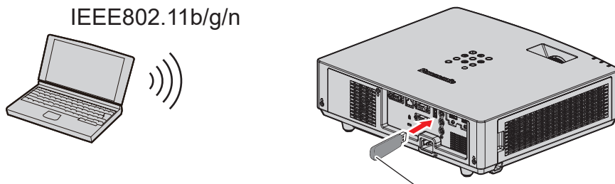
옵션 제공되는 액세서리의 무선 모듈 (모델번호: AJ-WM50)
