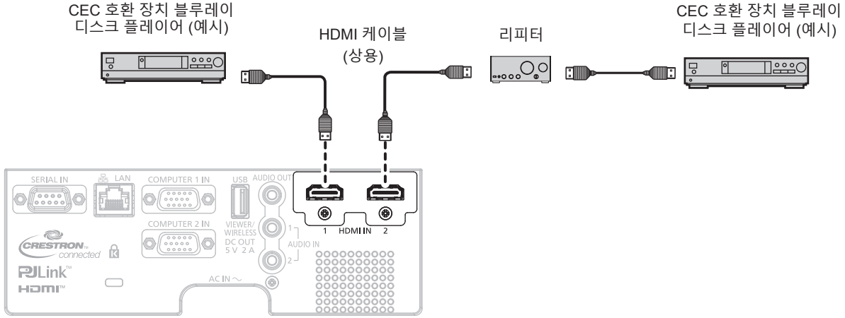
CEC 호환 장치와의 연결 예
