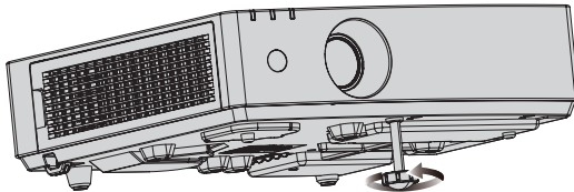
최대 조절 가능 범위 조절식 발: 30 mm (1-3/16")
