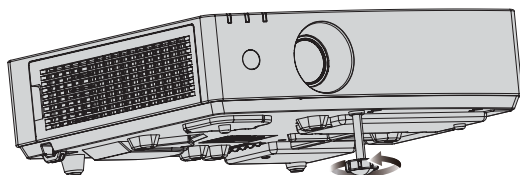
Максимальный диапазон настройки Регулируемая ножка 30 mm (1-3/16")
