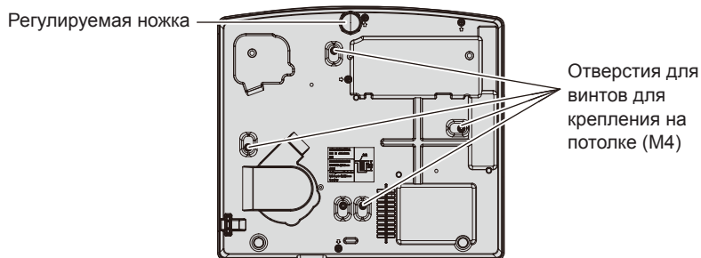
Положения отверстий для винтов для крепления на потолке и Регулируемая ножка
