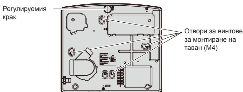
Позиции на отворите за винтове за таванен монтаж и регулируемия крак
