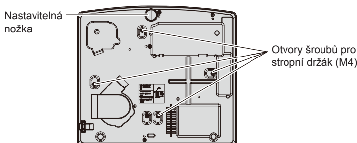
Polohy otvorů se závitem pro stropní upevňovací držák a poloha nastavitelná nožka
