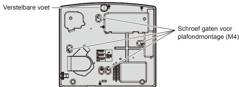
Posities van schroefgaten voor plafondmontage en verstelbare voet
