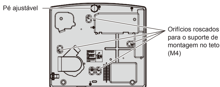
Posição dos orifícios de parafuso para montagem no teto e pé ajustável
