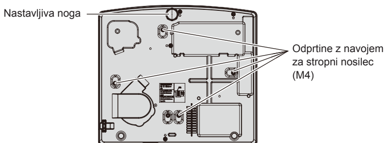
Položaji vrtin za stropno namestitev in nastavljiva noga
