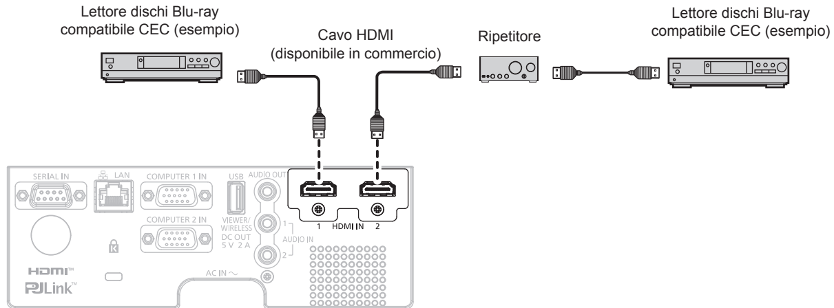
Esempio di connessione con dispositivo compatibile CEC
