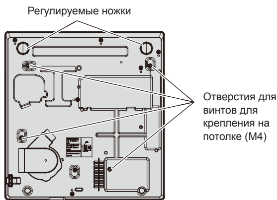
Положения отверстий для винтов для крепления на потолке и регулируемых ножек
