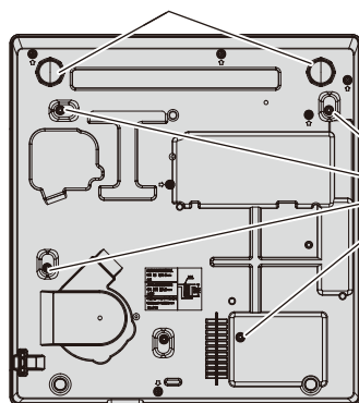
Skruehullernes positioner til loftsmontering og justerbare fødder
