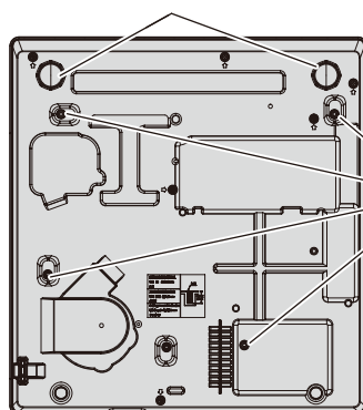
Położenie gwintowanych otworów do montażu uchwyty do mocowania na suficie oraz regulowanych stopek.
