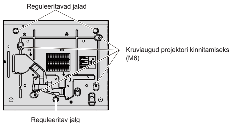
Reguleeritavate jalgade ja projektori kinnitamise kruviaukude asendid
