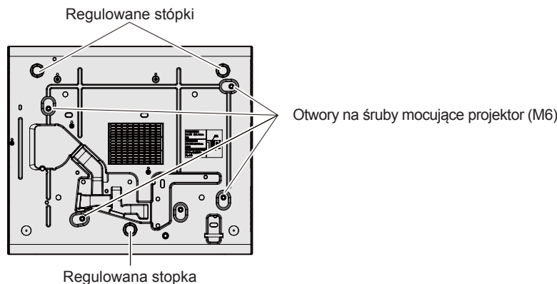
Położenie regulowanych stopek i otworów na śruby mocujące projektor
