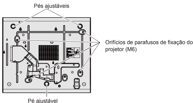
Posições dos pés ajustáveis e orifício de parafusos de fixação do projetor
