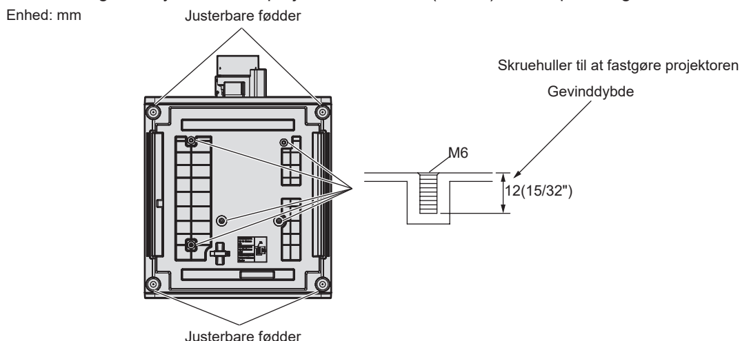
Skruehullernes positioner til fastgøring af projektoren og justerbare fødder
