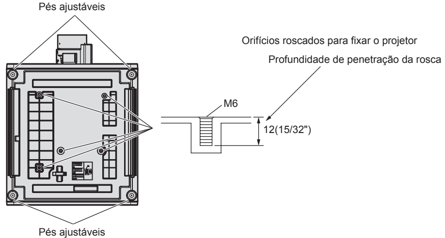
Posições dos orifícios roscados para fixar o projetor e os pés ajustáveis
