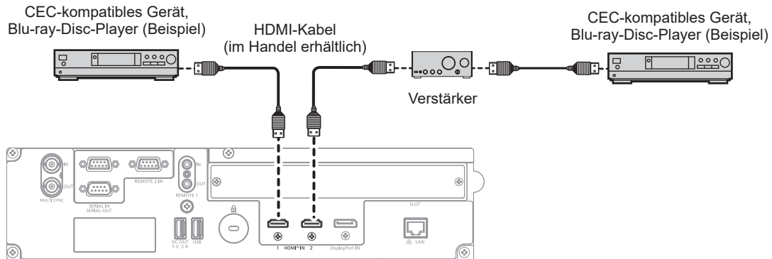
Anschlussbeispiel für ein CEC-kompatibles Gerät
