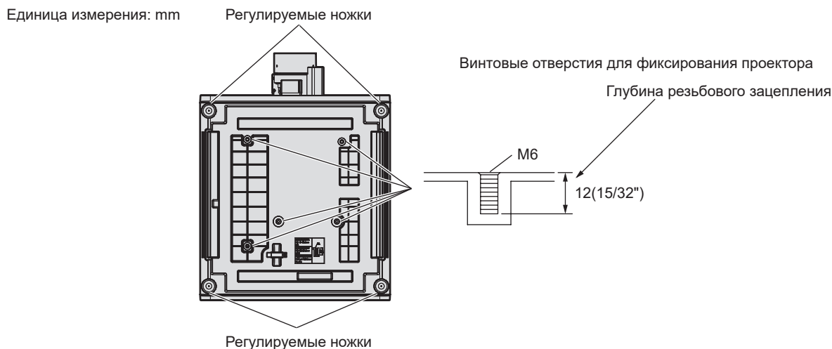
Положения отверстий для винтов для фиксирования проектора и регулируемых ножек
