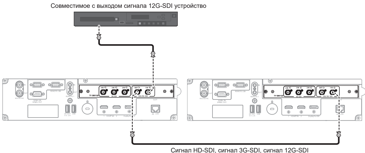
Сигнал HD-SDI, сигнал 3G-SDI, сигнал 12G-SDI
