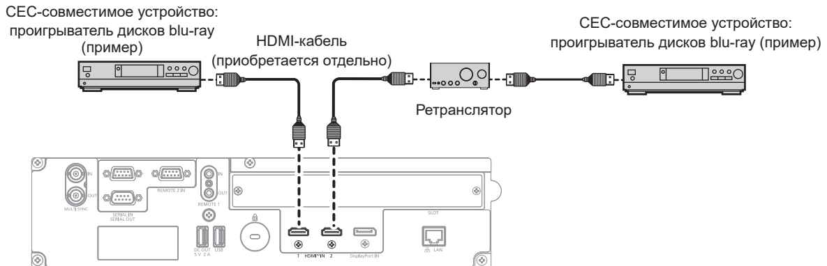
Пример подключения CEC-совместимого устройства
