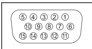
Disposizione dei piedini per il terminale di ingresso PC
