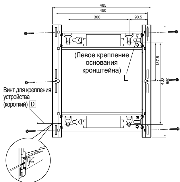
Вертикальная установка Единицы: мм
