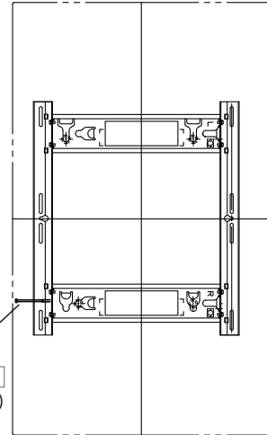
本体抜け防止用ねじ (短) D (締め付けトルクは 1.2 ~ 1.5 N・m)
