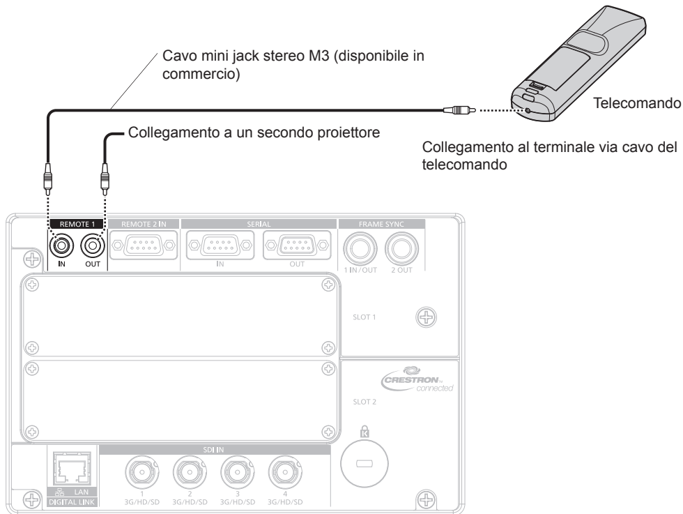
Terminali di collegamento
