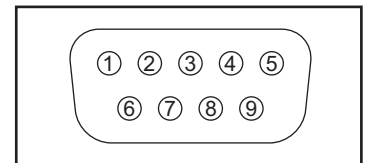
Stiftnummerung für die SERIAL-Buchse
