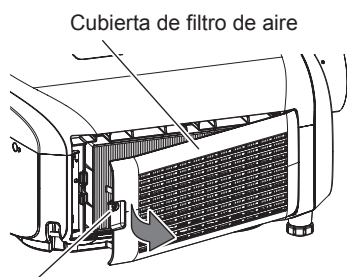
Tornillo de fijación de la cubierta de filtro de aire
