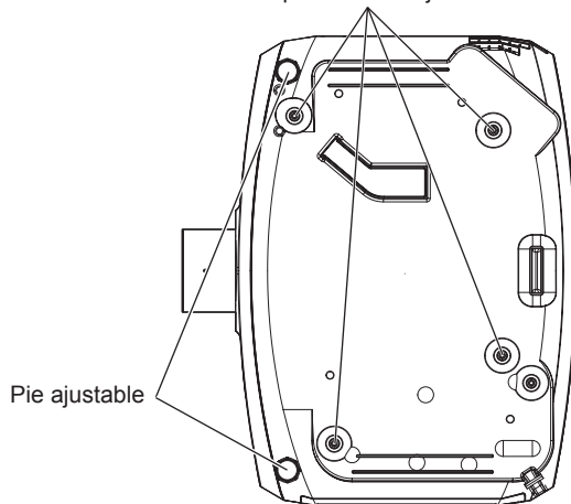
Posiciones de los orificios de tornillo para el montaje en el techo y uso de pie ajustable
