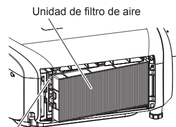
Compartimiento de la unidad de filtro de aire y orificio de entrada de aire del proyector
